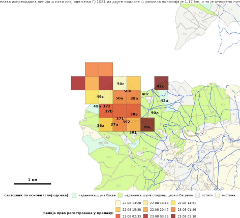
ПРЕШЕВО — ГДЕ ЈЕ КОНСТАТОВАН ПОЖАР, ПО ОДСЕЦИМА Келије од 375 m обојене по прелазу у коме су ПРВИ ГУТ регистроване: црне ознаке = одсеци у отisku (одељење+одсек) плава испрекидана линија = исти слој одељења ГЈ 1021 из друге подлоге — разлика положаја је 1,17 km, и то је отворено питање
